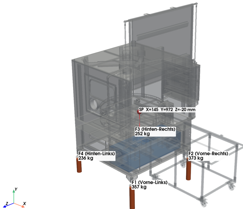
Abbildung 7. Fall C (Wasser + 300 kg Korblast, 1.218 kg).
