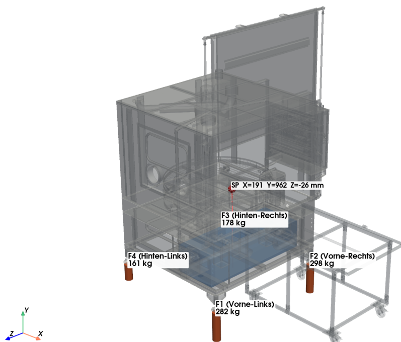
Abbildung 6. Fall B (Tank gefüllt, 918 kg): Das Wasservolumen ist als blauer Quader dargestellt.
