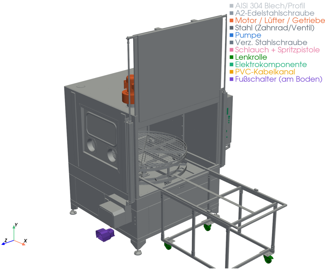
Abbildung 1. 3D-Ansicht der Baugruppe, nach Werkstoffklassen eingefärbt (grau: AISI 304 Blech/Profil).
