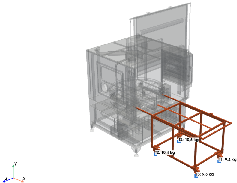
Abbildung 11. Beladewagen C011459 (39,7 kg) — eigene Rollenlasten T1-T4; keine Last auf den Maschinenfüßen.
