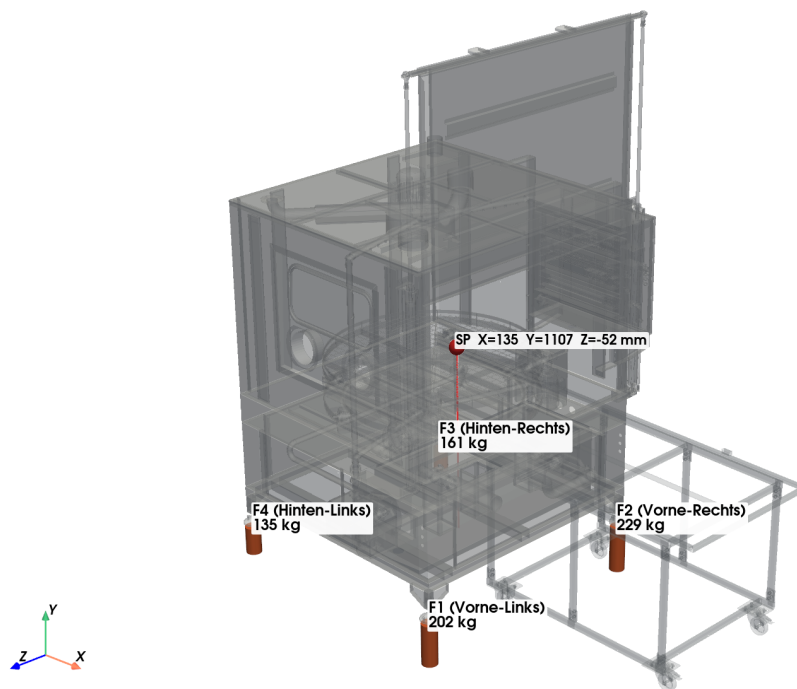
Abbildung 5. Fall A (trockene Maschine, 727 kg): SP-Lage und Fußlasten; die Höhe der orangenen Zylinder ist proportional zur Last.
